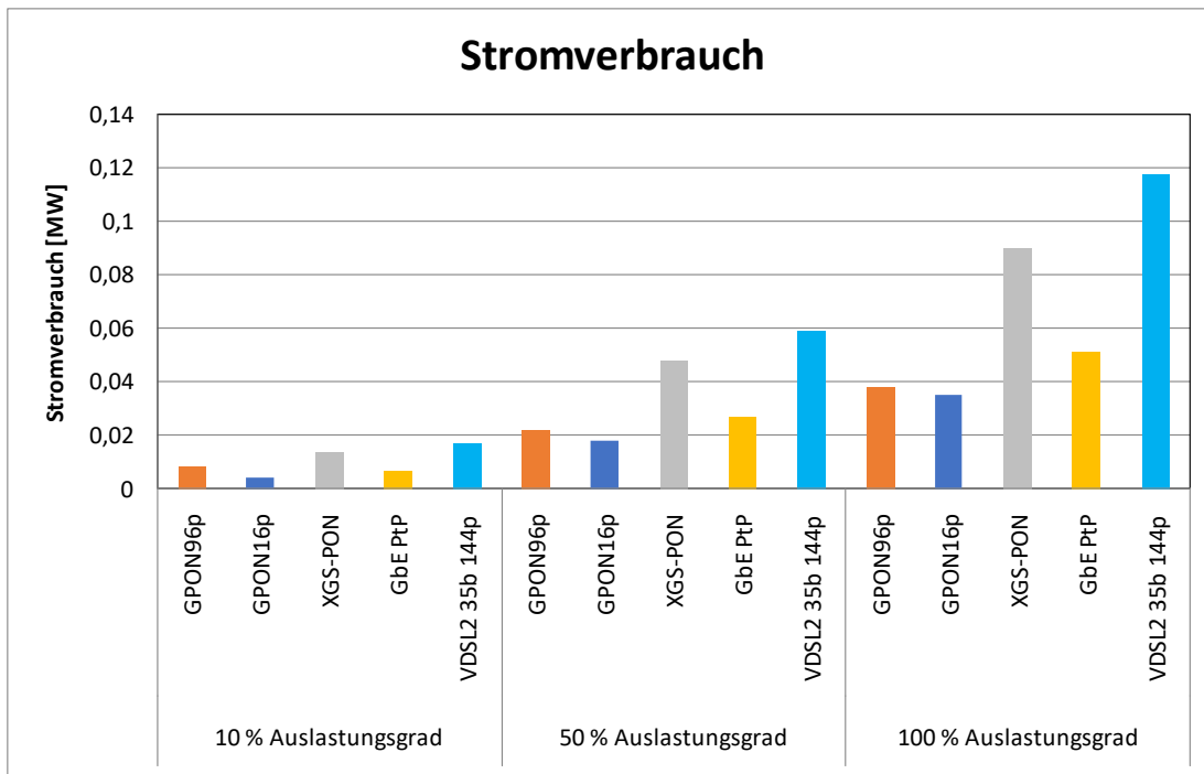
ABBILDUNG 19: STROMVERBRAUCH FÜR EINE VERSORGUNG VON HALTERN AM SEE MIT DER JEWEILIGEN ZUGANGSNETZTECHNOLOGIE FÜR VERSCHIEDENEN AUSLASTUNGSGRAD.
