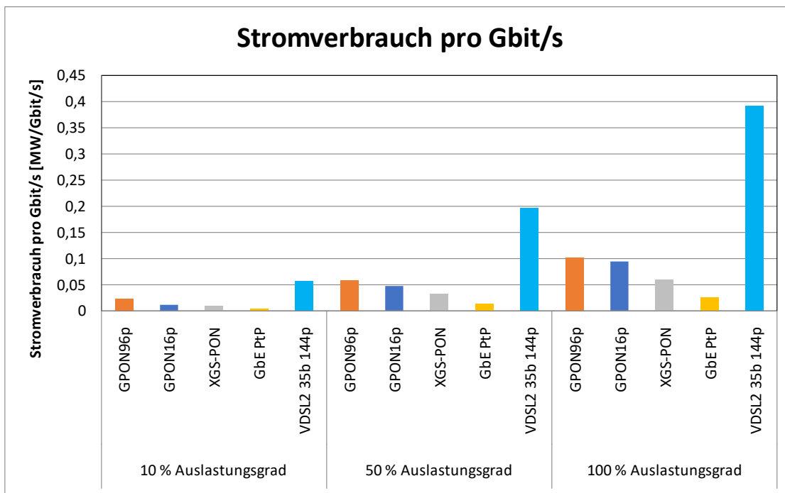
ABBILDUNG 20: STROMVERBRAUCH PRO GBIT/S FÜR EINE VERSORGUNG VON HALTERN AM SEE MIT DER JEWEILIGEN ZUGANGSNETZTECHNOLOGIE FÜR VERSCHIEDENEN AUSLASTUNGSGRAD.
